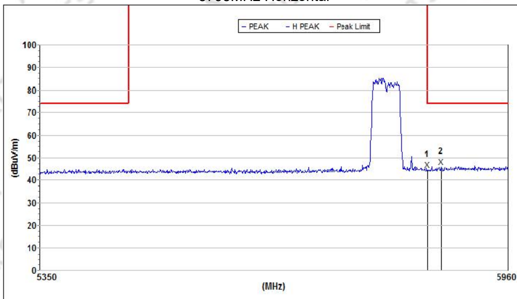
5795MHz Horizontal
