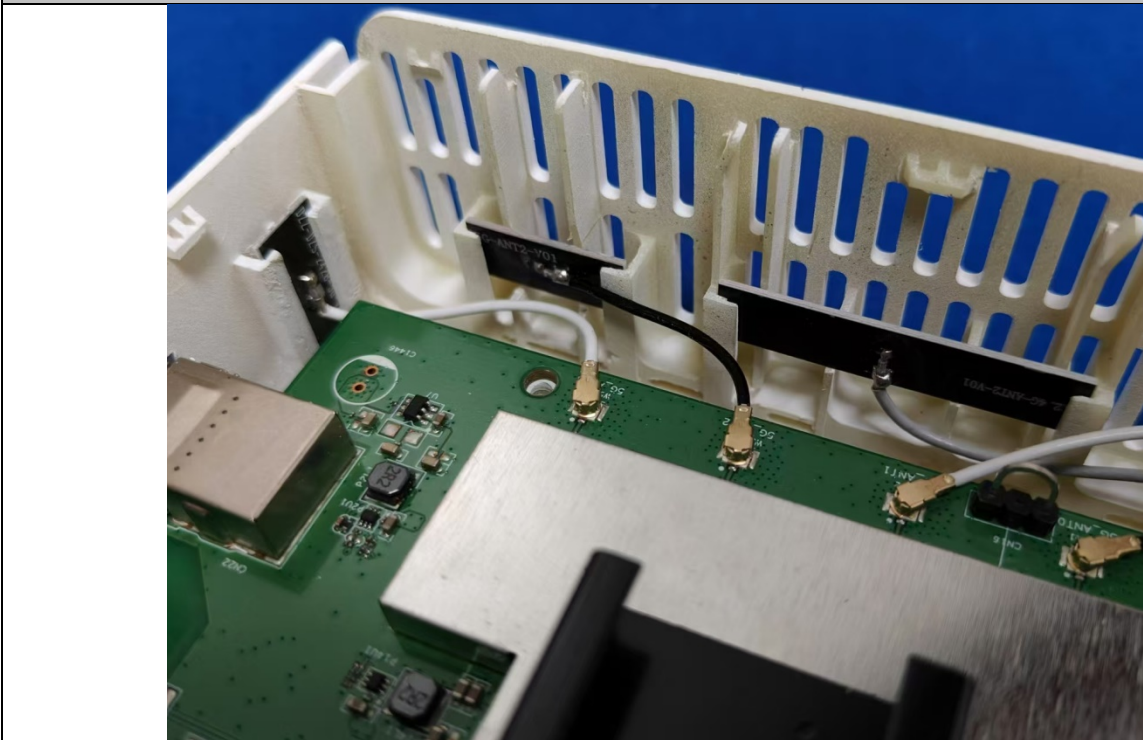
EUT Photo
