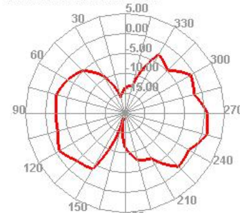
5850.000MHz E2
