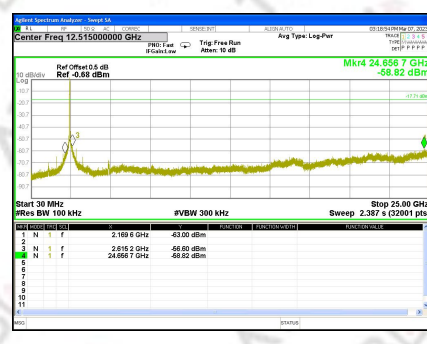
CH9_Ant. 0
