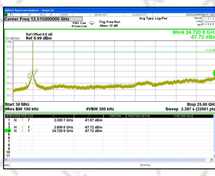
CH6_Ant. 0
