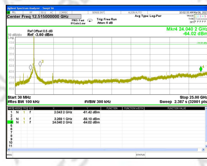
CH9_Ant. 1
