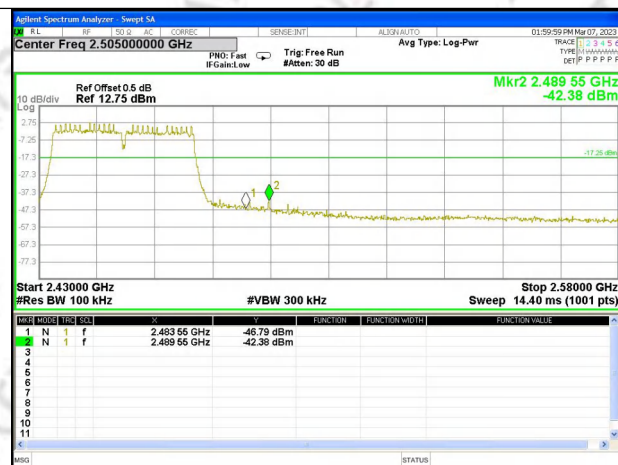
CH9_Ant. 0
