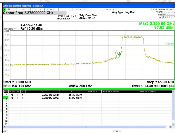
CH1_Ant. 0
