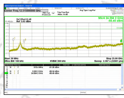
CH11Ant. 1
