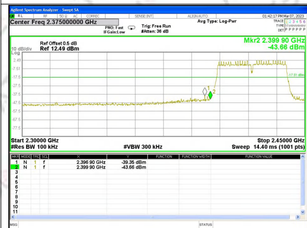
CH3_Ant. 0
