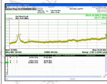
CH3_Ant. 0
