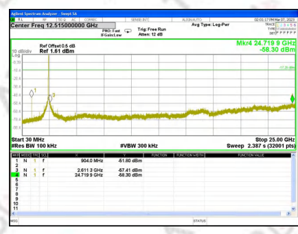
CH9_Ant. 0
