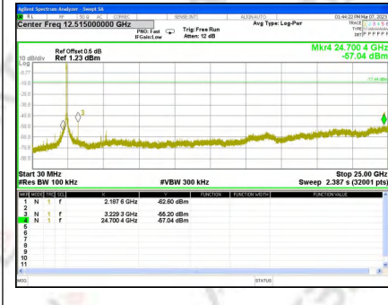
CH3_Ant. 1
