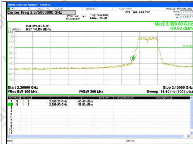
CH1_Ant. 1
