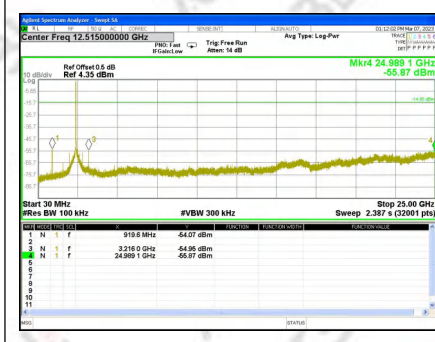
802.11ac40_MIMO
