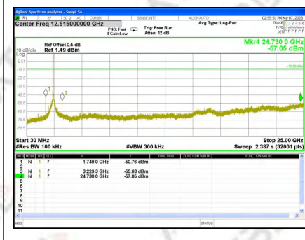
802.11ac20
