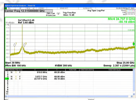
CH11Ant. 1
