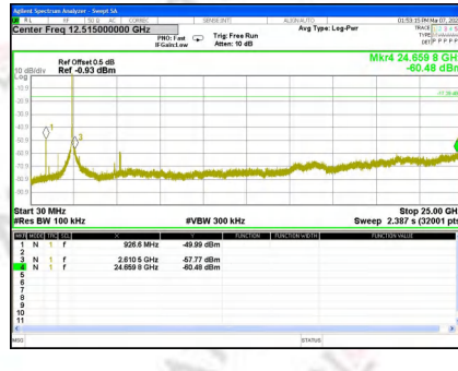
CH6_Ant. 1
