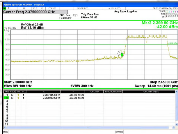
CH3_Ant. 1
