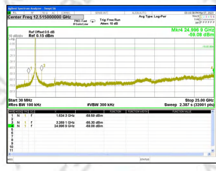
CH9_Ant. 1
