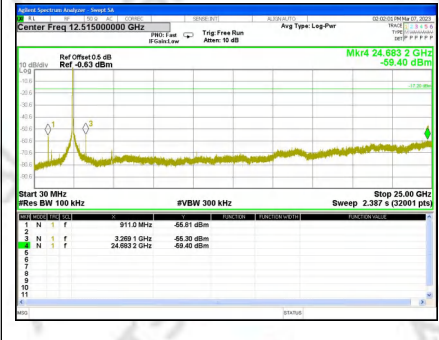
CH9_Ant. 1
