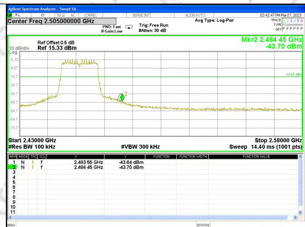
CH11_Ant. 0
