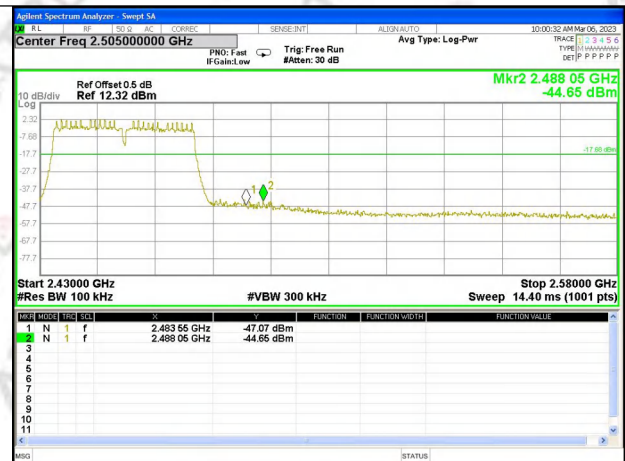
CH9_Ant. 1
