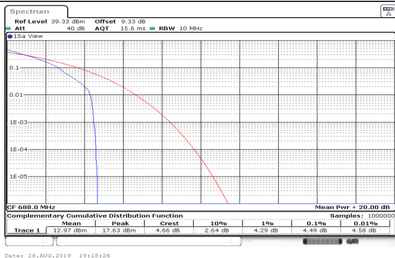
Band71-20MHz-QPSK-133372-100RB#0
