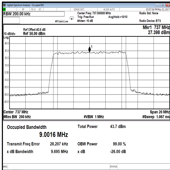
16QAM / RxTx1
