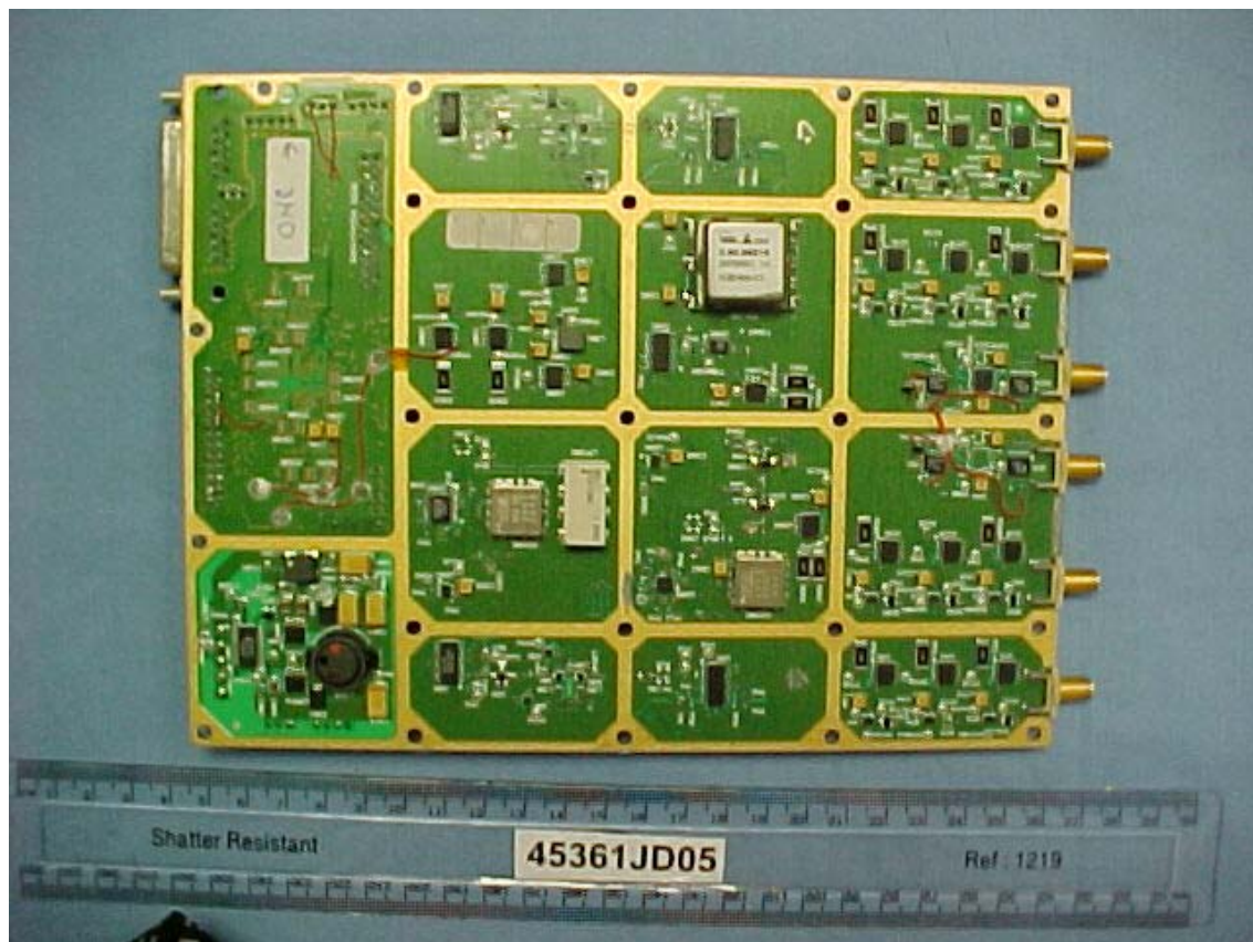
DZ PCB1 Side 2
