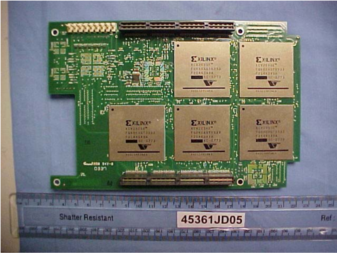
DN PCB1 Side 2
