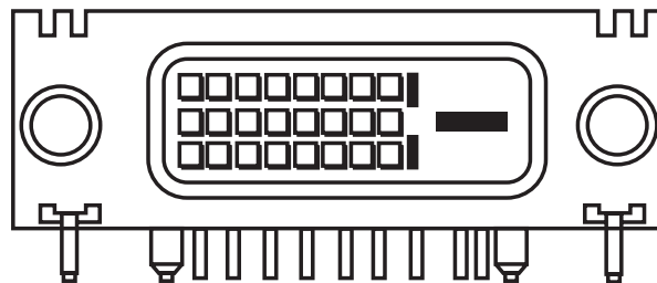
D-SUB DRAWING(CN10)
