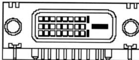
D-SUB DRAWING(CN10)
