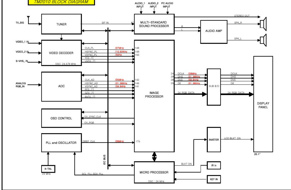
TM2010 BLOCK DIAGRAM
