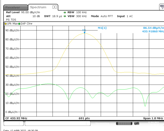
Plot 2 – OOK modulation
