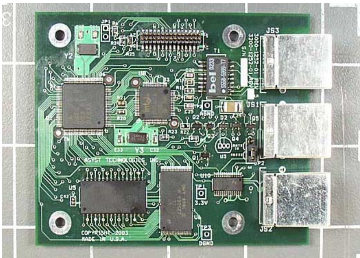
PCB 2 Top
