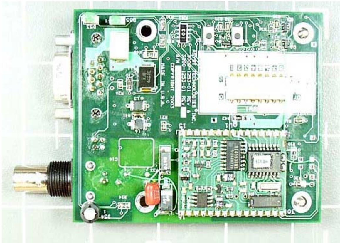
PCB 1 Bottom
