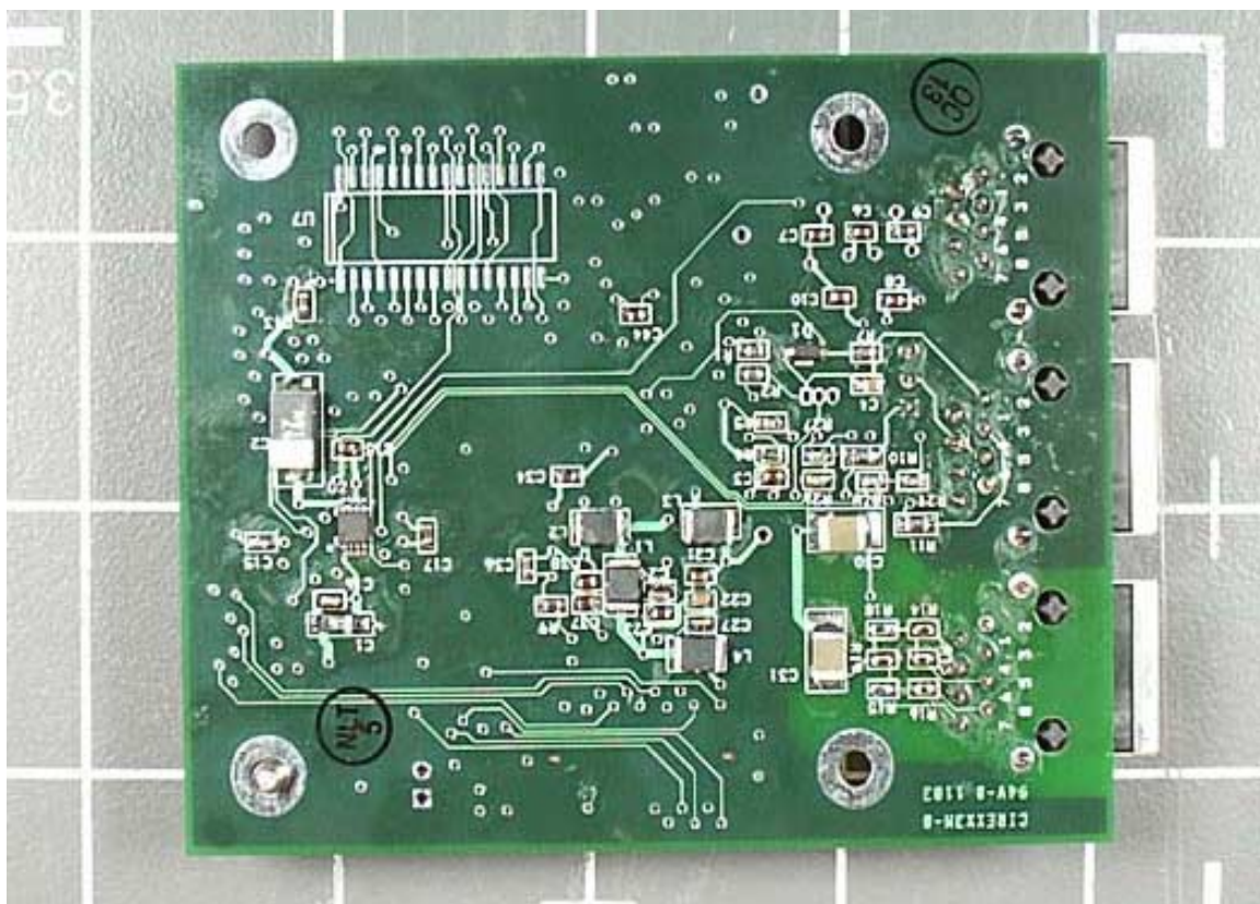
PCB 2 Bottom
