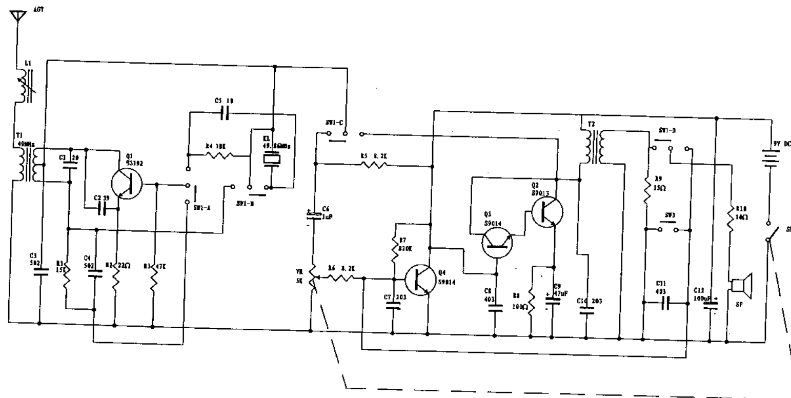
對講機線路圖
