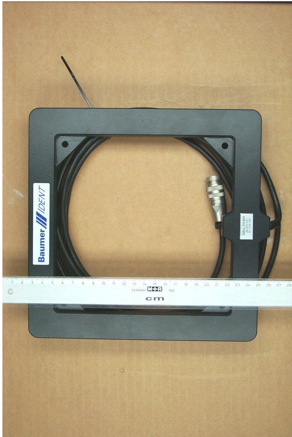
20382_5.jpg OISL 77LA04/2-SER antenna type OIS-L 77LS03
