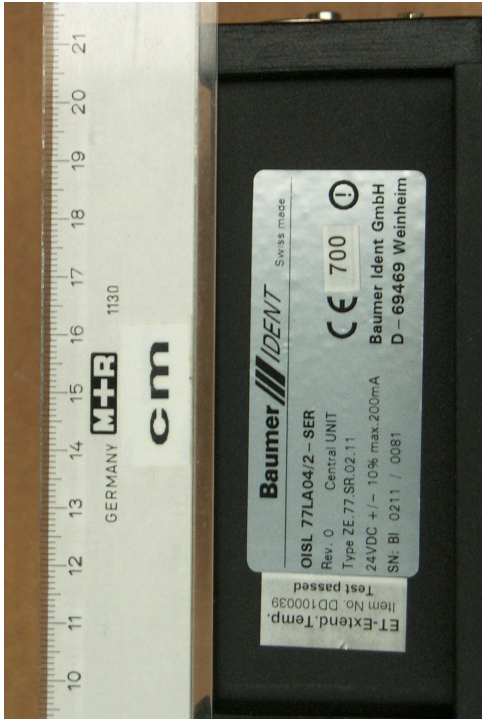
20382_1.jpg OISL 77LA04/2-SER type plate
