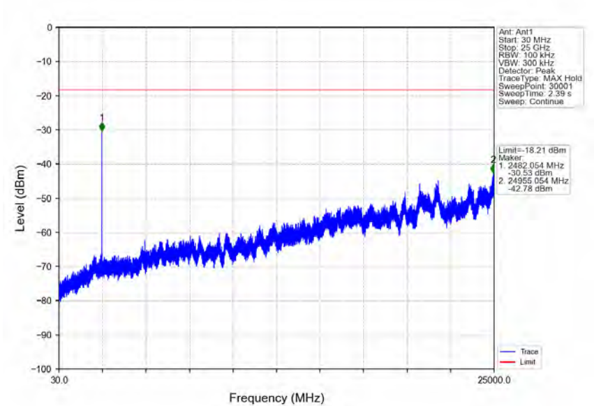
2M_HCH_2480MHz_Ant1_NTNV
