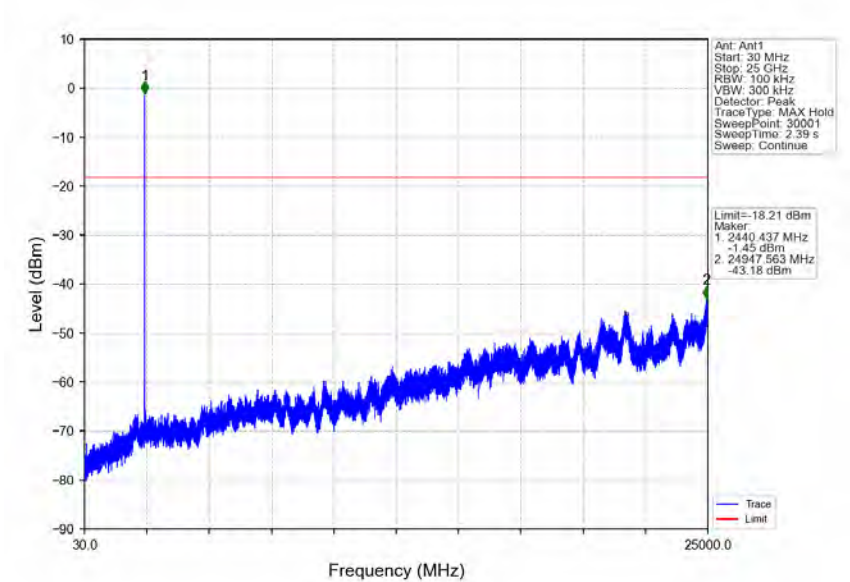
2M_MCH_2440MHz_Ant1_NTNV
