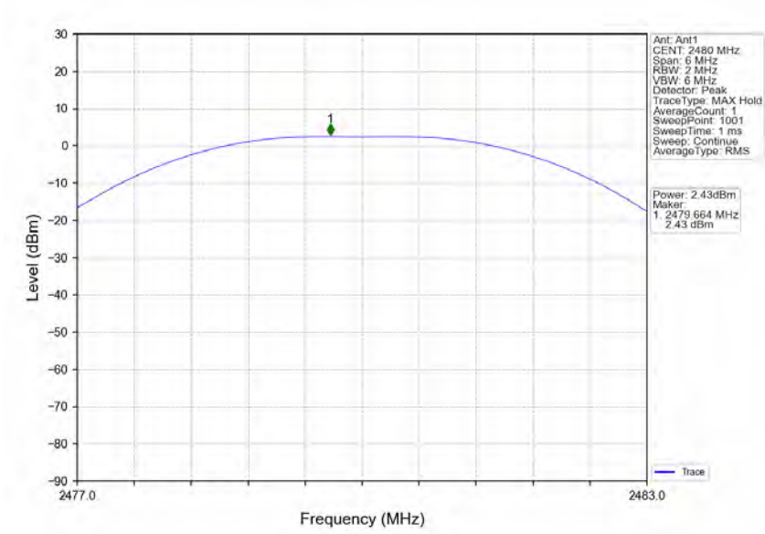
2M_HCH_2480MHz_Ant1_NTNV
