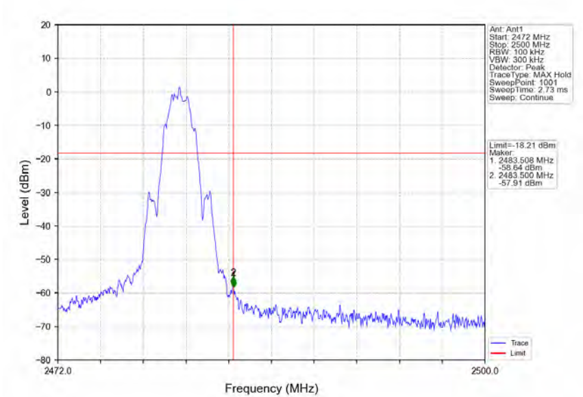
2M_HCH_2480MHz_Ant1_NTNV
