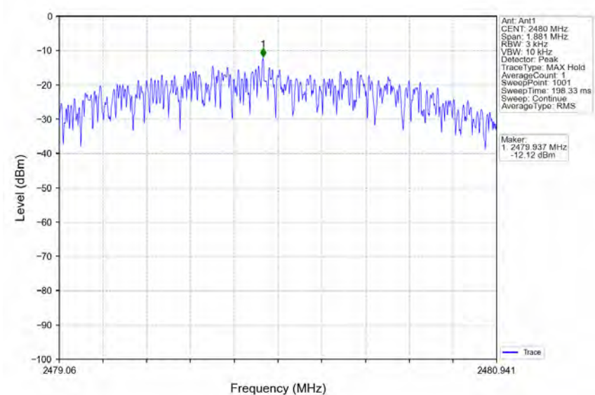
2M_HCH_2480MHz_Ant1_NTNV
