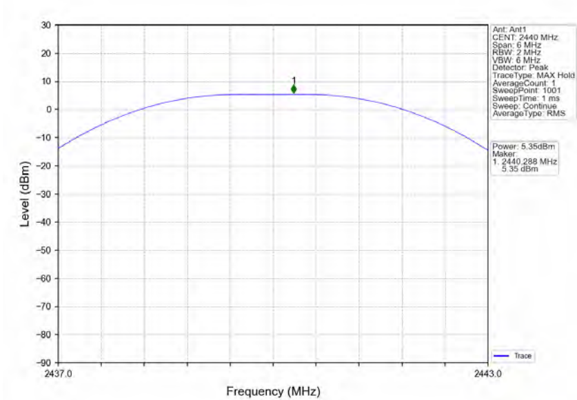
2M_MCH_2440MHz_Ant1_NTNV
