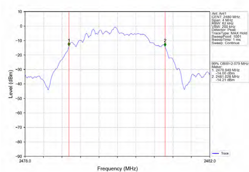
2M_HCH_2480MHz_Ant1_NTNV
