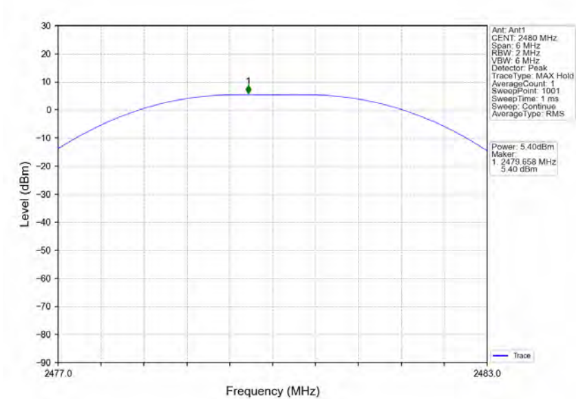
2M_HCH_2480MHz_Ant1_NTNV
