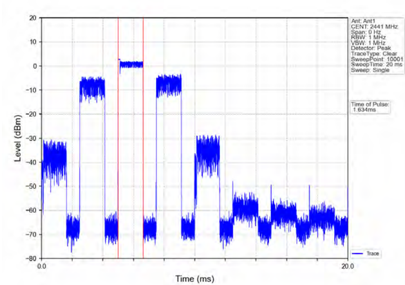
Pi/4DQPSK_2DH3_HOPP_Ant1_NTNV
