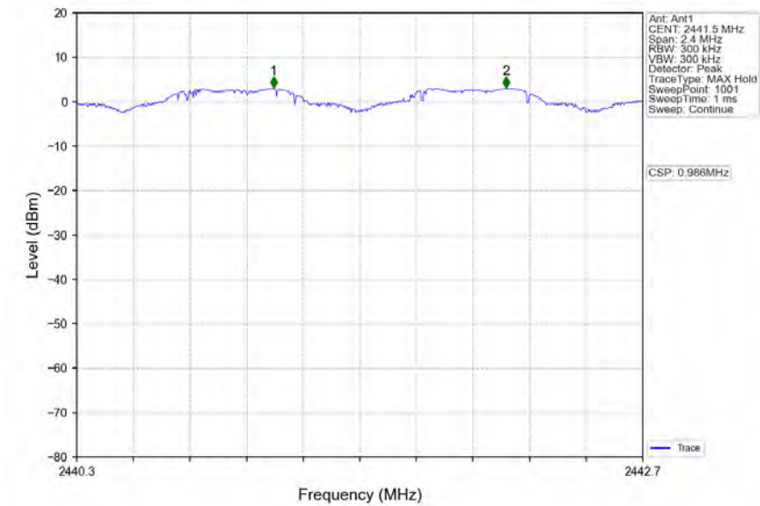
8DPSK_3DH5_HOPP_Ant1_NTNV
