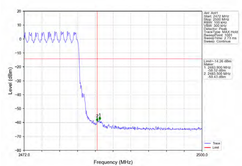
Pi/4DQPSK_2DH5_HOPP_Ant1_NTNV
