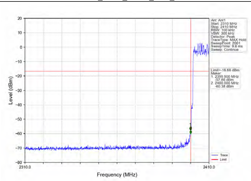
Pi/4DQPSK_2DH5_HOPP_Ant1_NTNV
