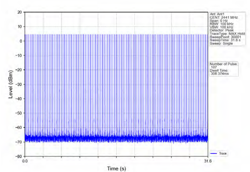
GFSK_DH5_HOPP_Ant1_NTNV
