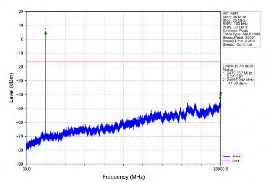
GFSK_DH5_HOPP_Ant1_NTNV
