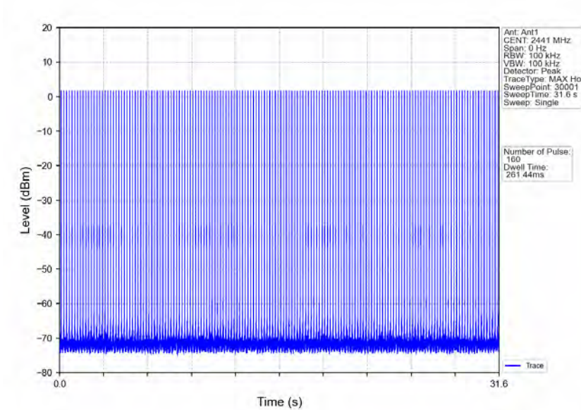
Pi/4DQPSK_2DH3_HOPP_Ant1_NTNV
