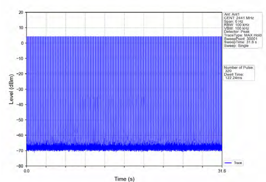
Pi/4DQPSK_2DH1_HOPP_Ant1_NTNV
