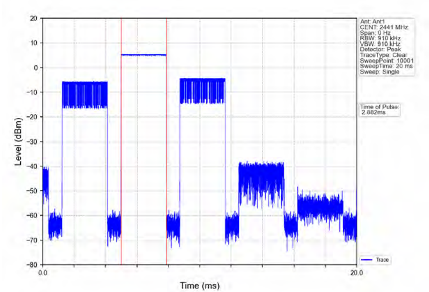
GFSK_DH5_HOPP_Ant1_NTNV
