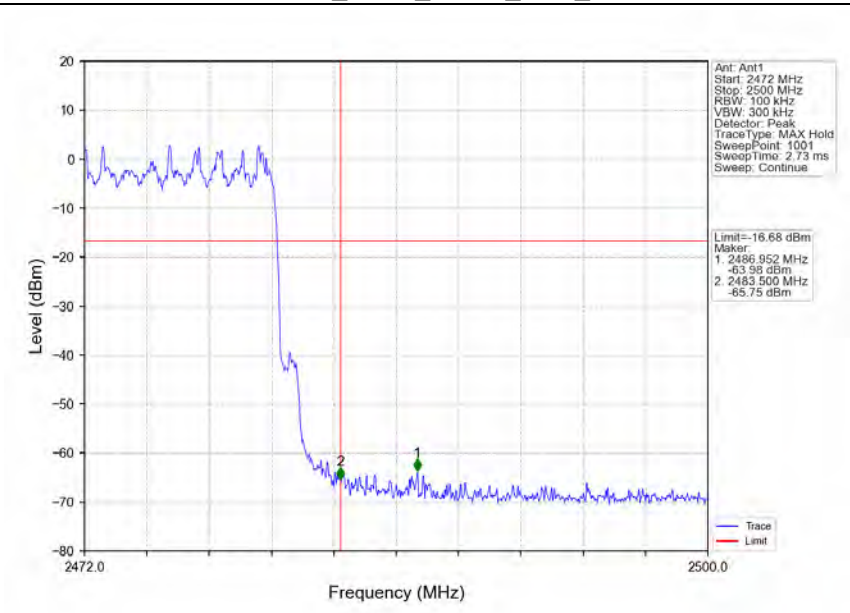
Pi/4DQPSK_2DH5_HOPP_Ant1_NTNV
