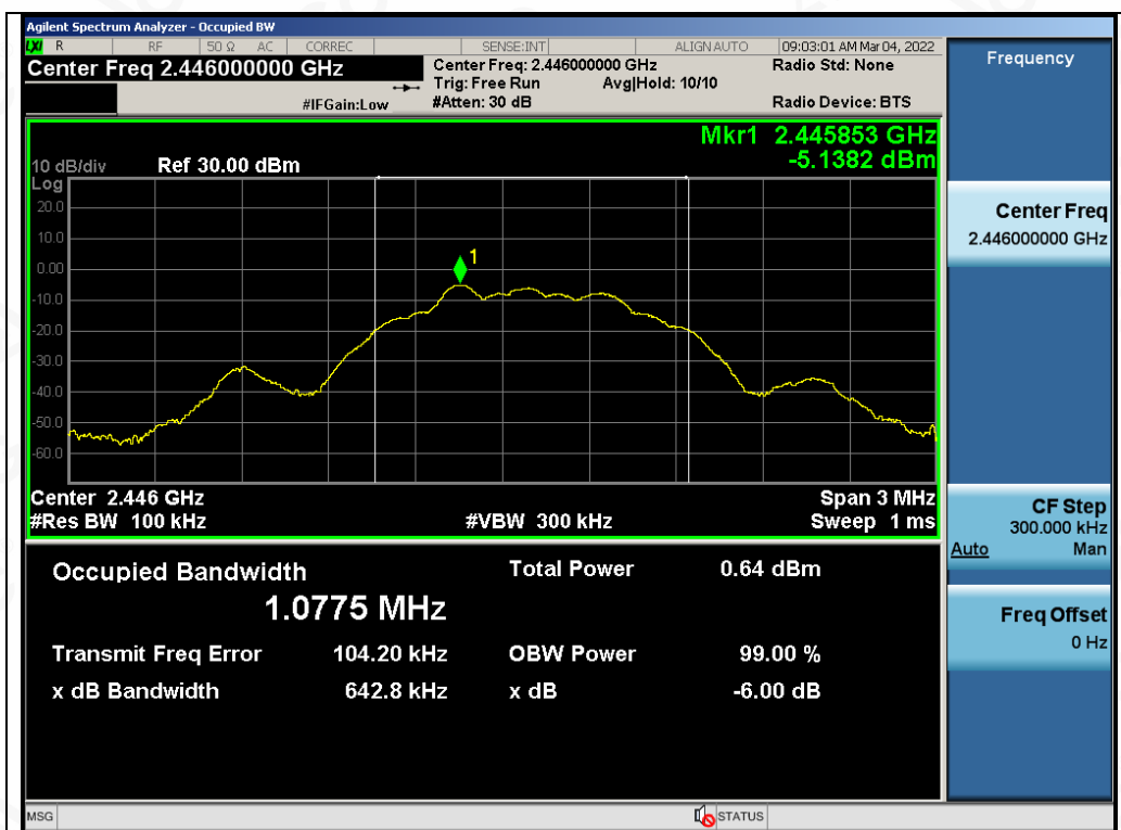
Test_Graph_GFSK_ANT1_2446_DTSBW
