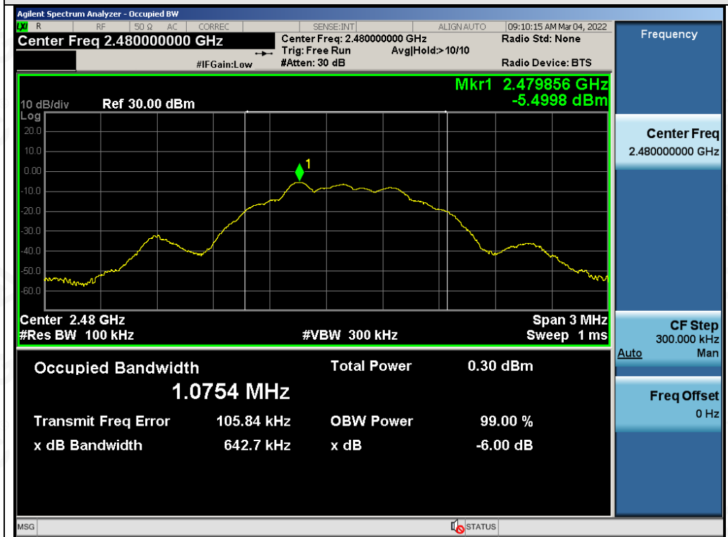
Test_Graph_GFSK_ANT1_2480_DTSBW
