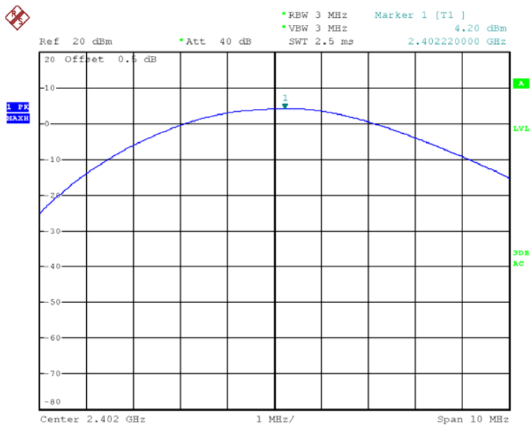
BLE Low Channel
