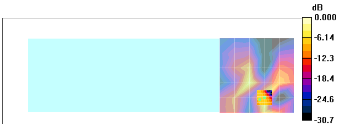
Radial/Longitudinal, GSM1900
