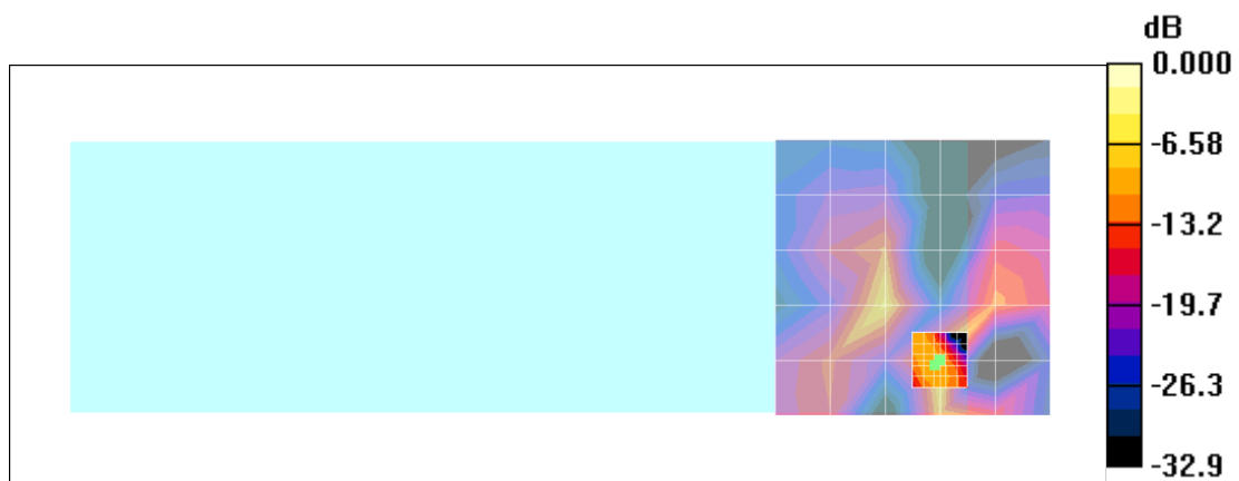
Radial/Longitudinal, GSM850
