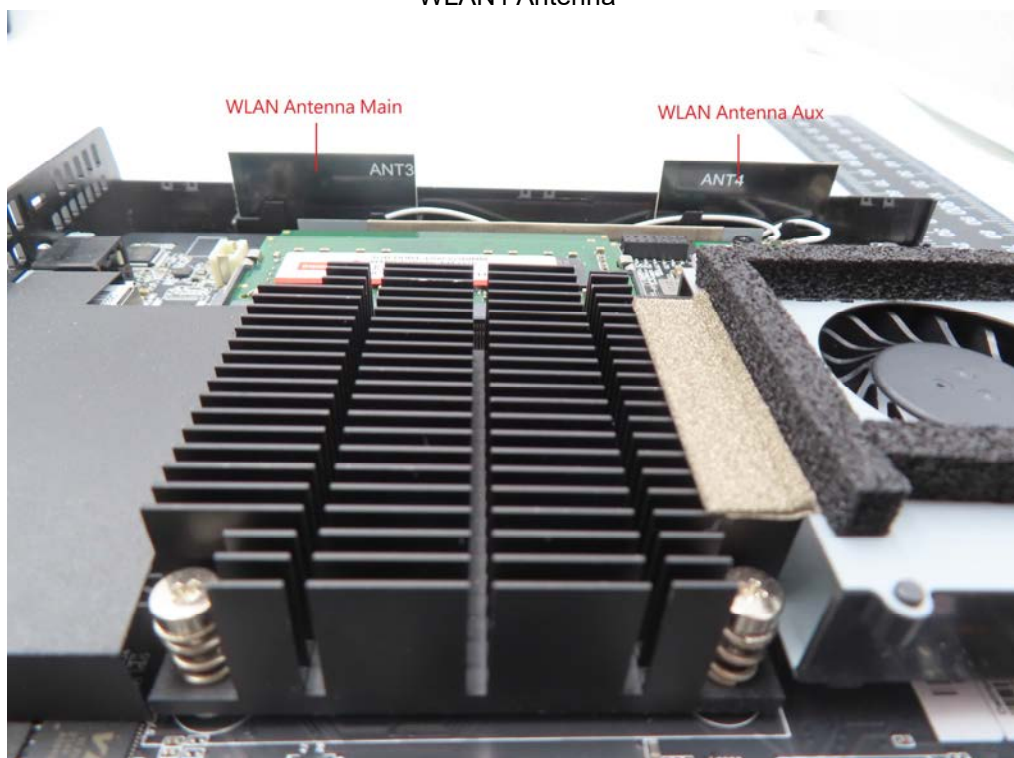
WLAN1 Antenna
