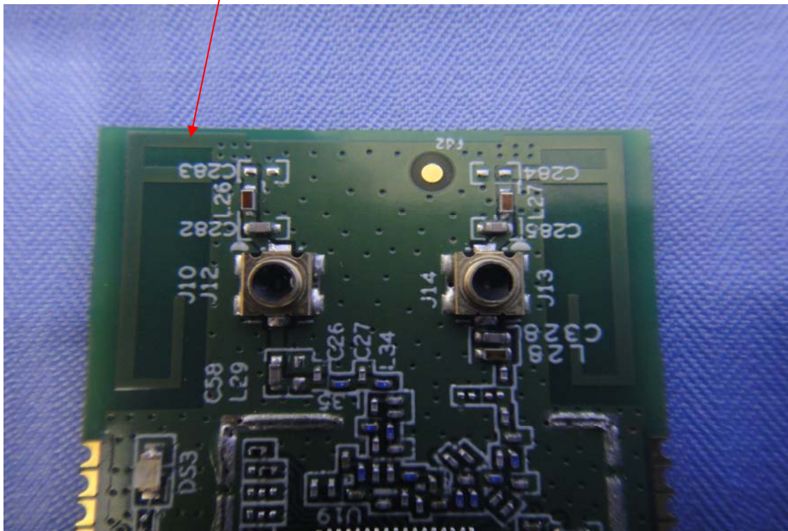
PIFA Antenna
