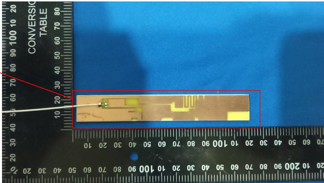
PIFA Antenna (Antenna 2)
