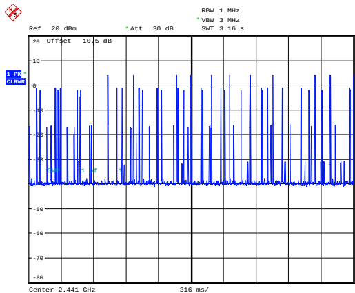
2EDR_DH5_Hopping
