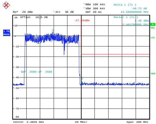
3EDR_DH1_Hopping_Upper
