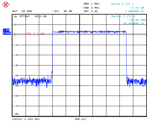
2EDR_DH3_Hopping
