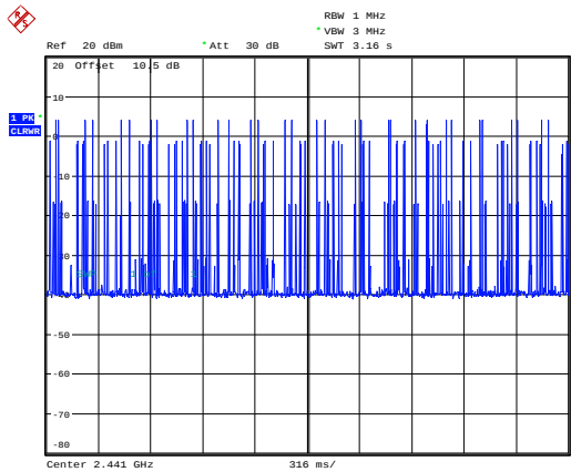
2EDR_DH1_Hopping
