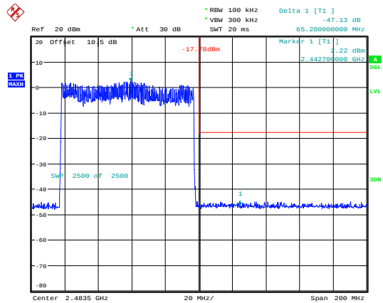
2EDR_DH1_Hopping_Upper
