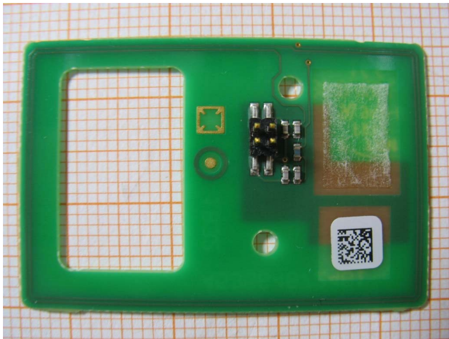
Photo 4: EUT
