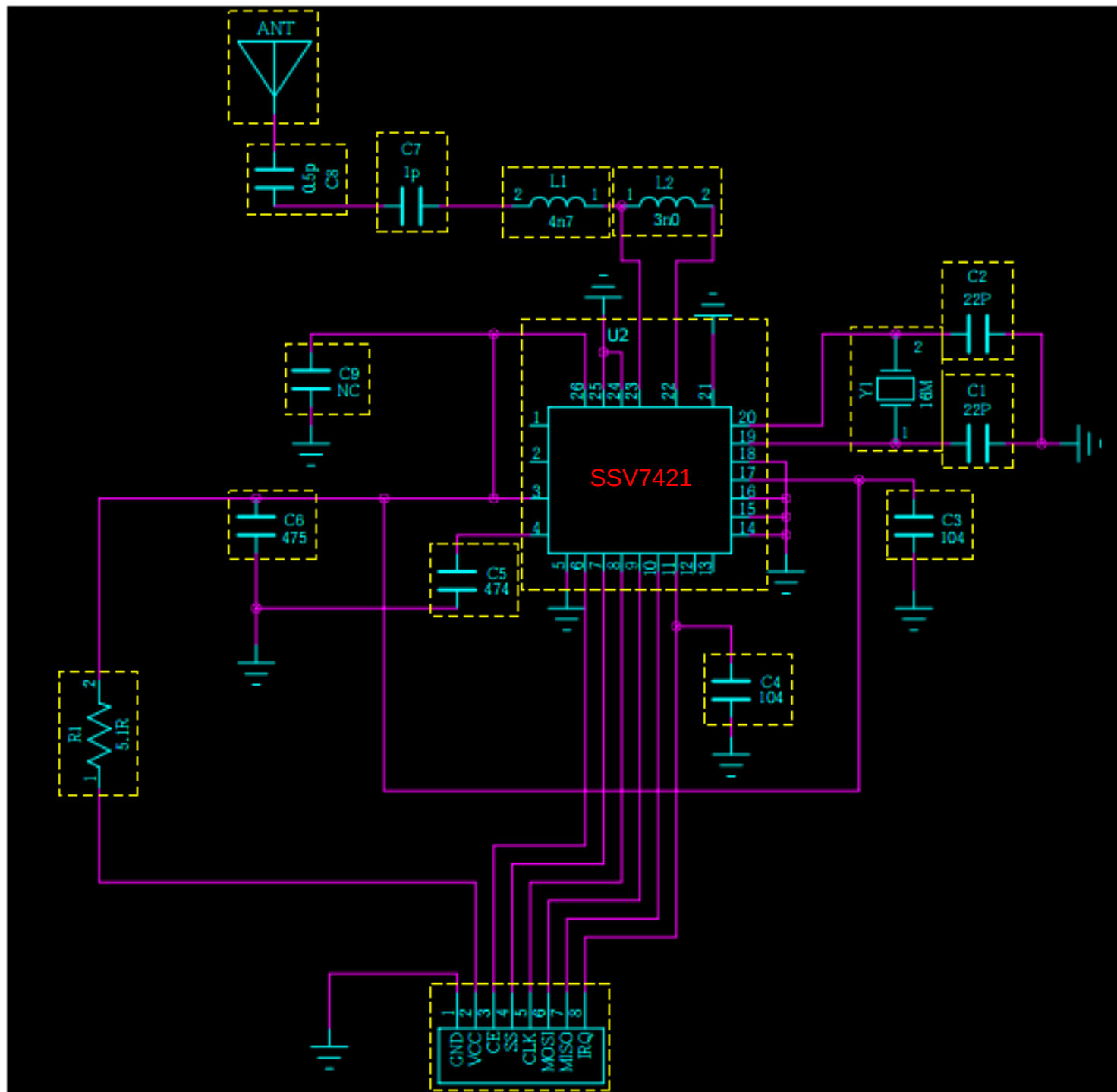
RF Module WT24DK2015A
