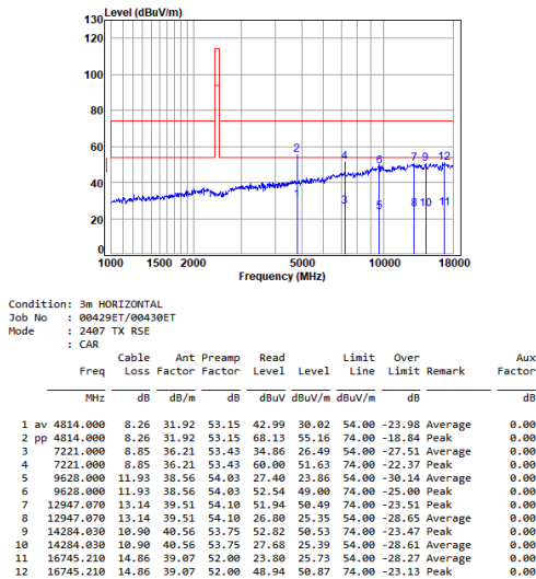
2.4G_SRD_LOW_TX_Horizontal
