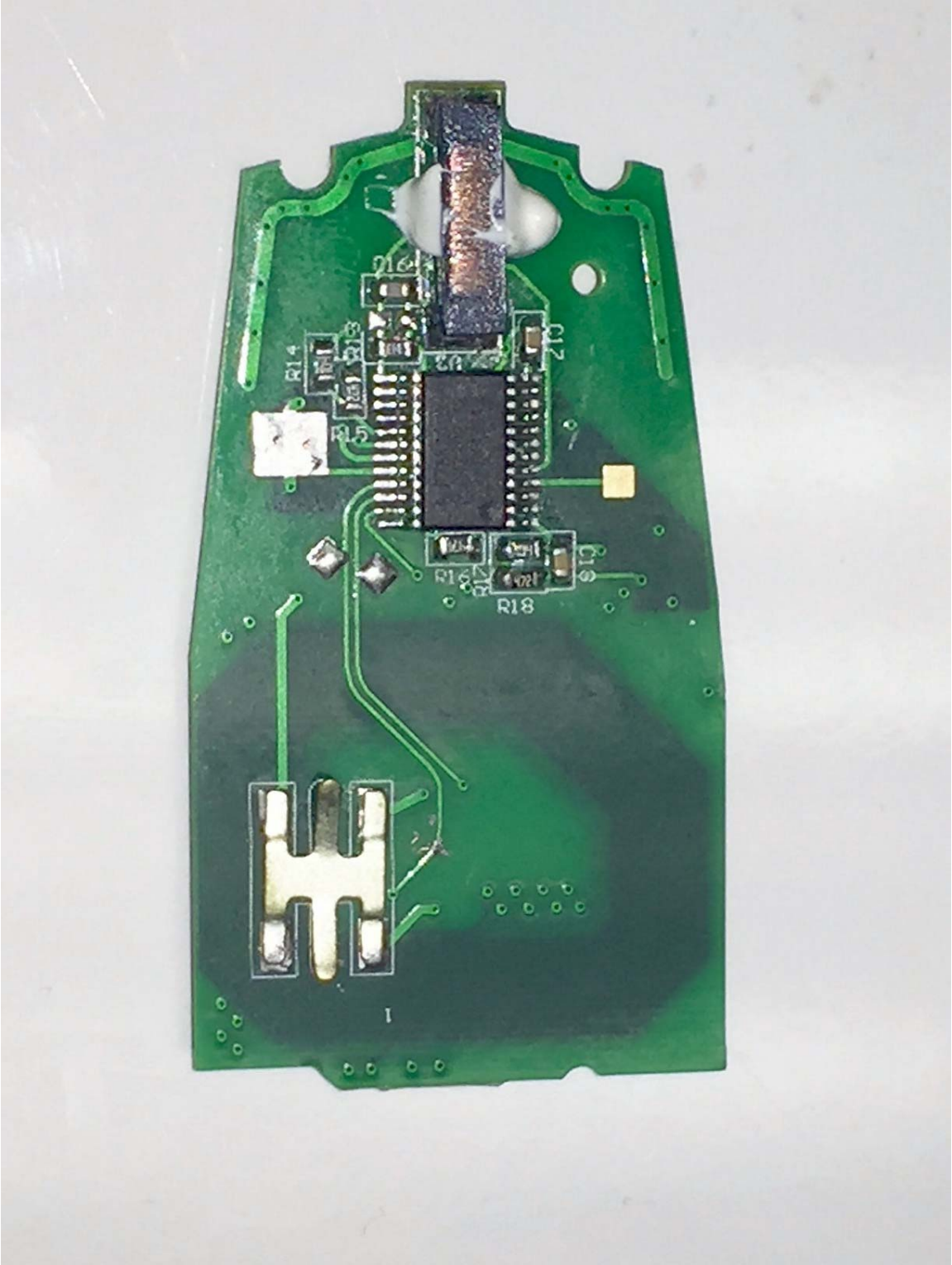
PCB Bottom
