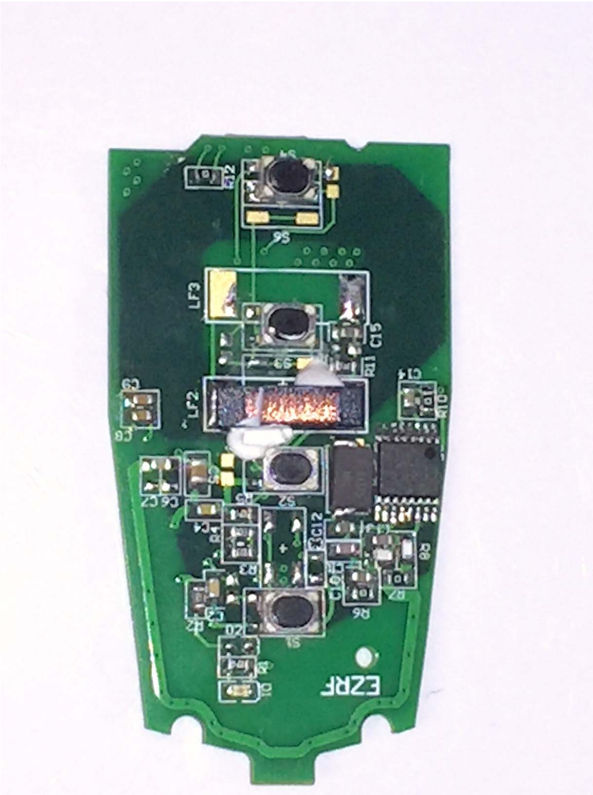
PCB Top
