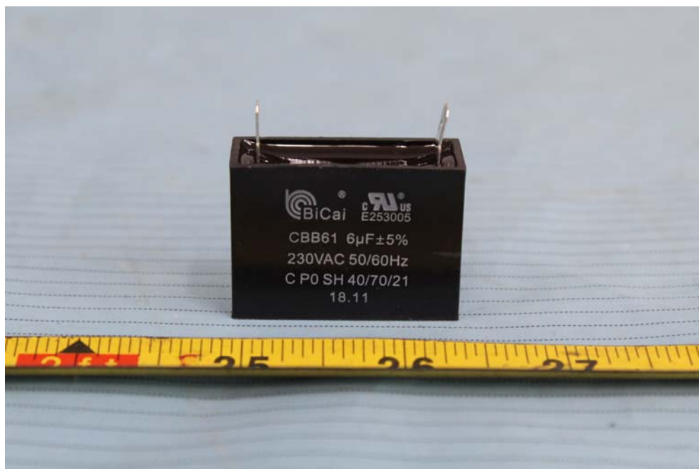
EUT –CBB61View
