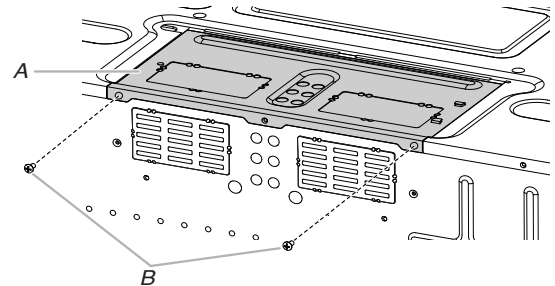
A. Placa de la compuerta B. Tornillos
