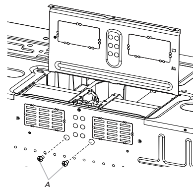
A. Tornillos del soplador (en orificios embutidos)
