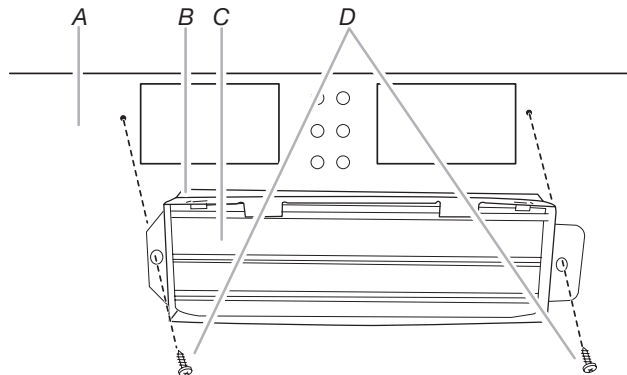
A. Parte posterior del horno de microondas B. Conjunto de la compuerta C. Hoja de la compuerta D. Tornillo para metal laminado #6 x 3/8"
