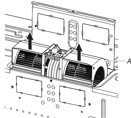
A. Moteur de ventilateur
