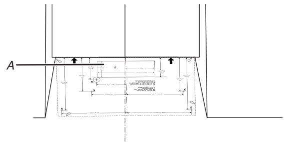
A. Zone de coupe pour l'évacuation par le mur
