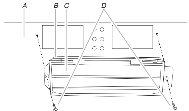
A. Face arrière du four à micro-ondes B. Module du clapet anti-reflux C. Lame du clapet anti-reflux D. Vis à tôle de 6 x 3/8 po (2)
