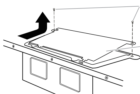
A. Screws B. Damper plate
