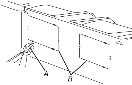
A. Alicata de corte diagonal para cable B. Cubiertas de ventilación de la compuerta
