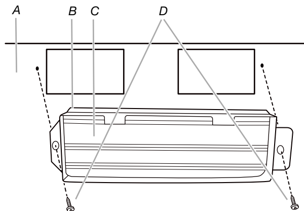
A. Arrière du four à micro-ondes B. Ensemble de registre C. Plaque du registre D. Vis à tôle de 5/32 po x 5/16 po (4 mm x 8 mm)
