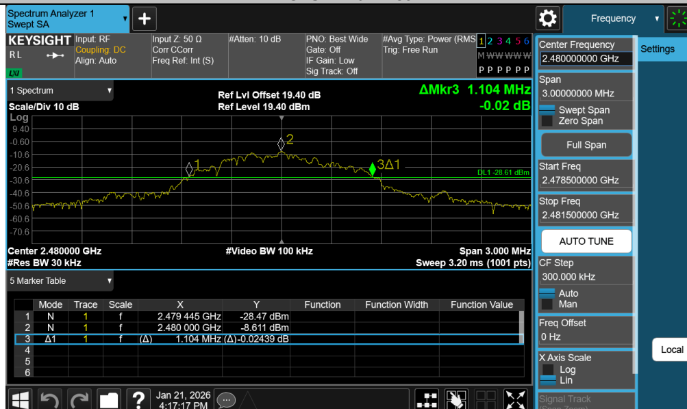
GFSK-Ant1-2480
