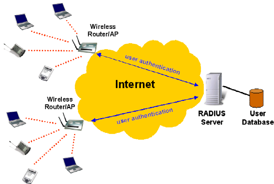
Fig. 52. IEEE 802.1x and RADIUS.
