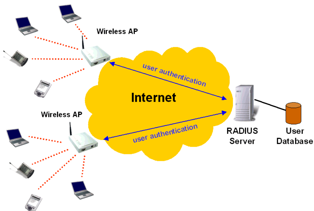
Fig. 52. IEEE 802.1x and RADIUS.
