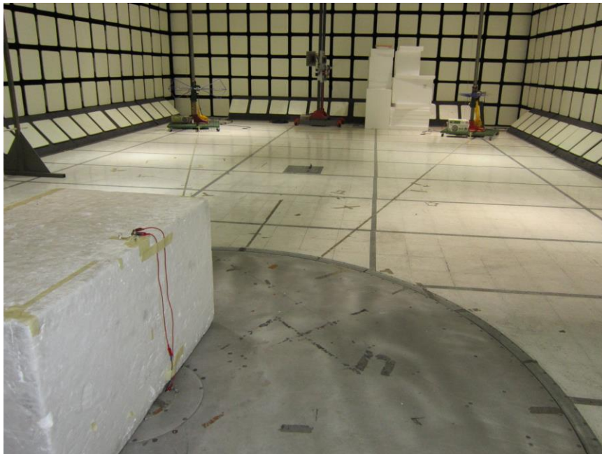
Below 1GHz EUT 80cm
