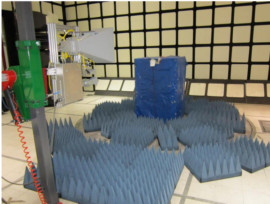
Above 1GHz EUT 1.5m
