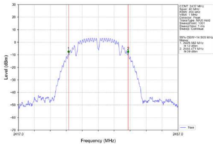
802.11b_MCH_2437MHz_Ant1 (SISO)_NTNV
