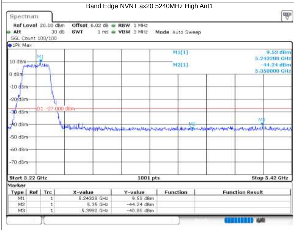
Band Edge NVNT ax20 5240MHz High Ant1
