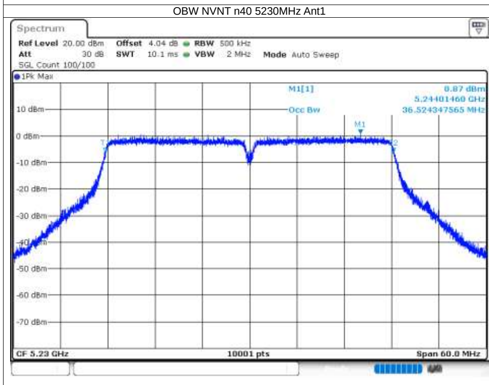
OBW NVNT n40 5230MHz Ant1
