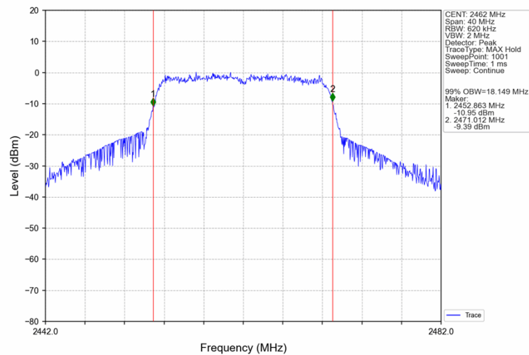
802.11n(HT20)_HCH_2462MHz_Ant2 (SISO)_NTNV
