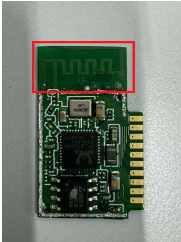
Antenna
