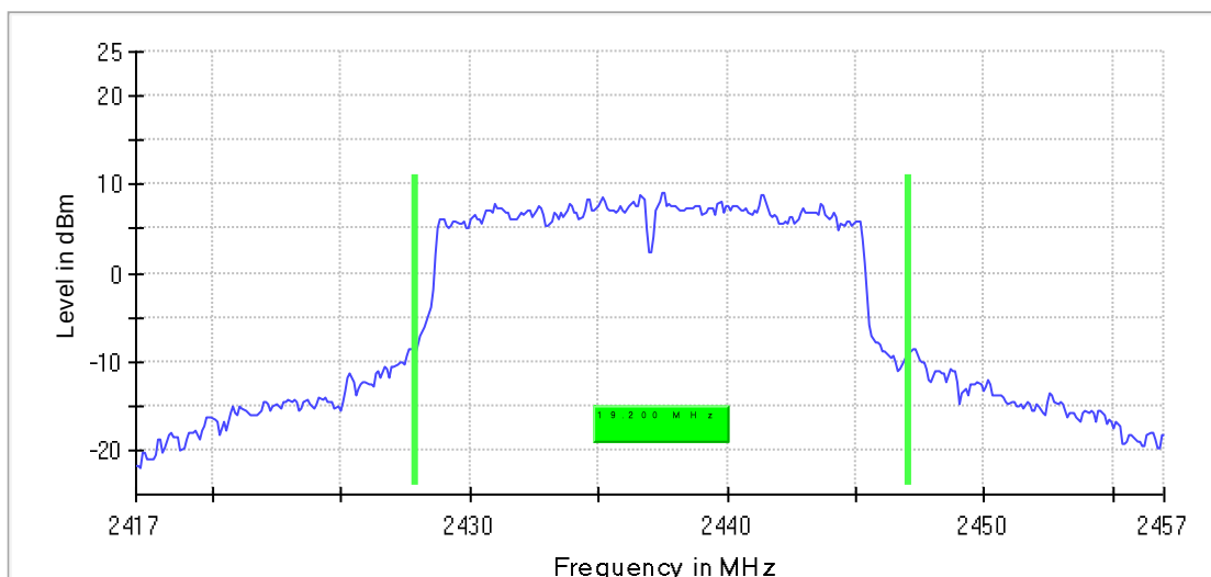
Mode 1 / CH6 (2437 MHz)
