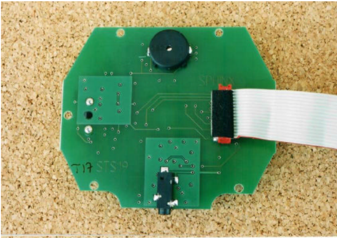
DMT 32 (TIRIS) – Face & PCB Back
