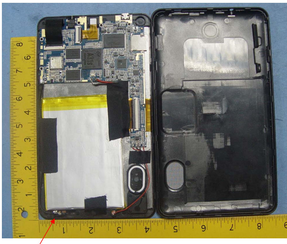
Antenna
