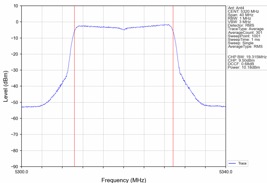
802.11ax(HEW20)_HCH_5320MHz_RU242_Left_Ant4_NTNV
