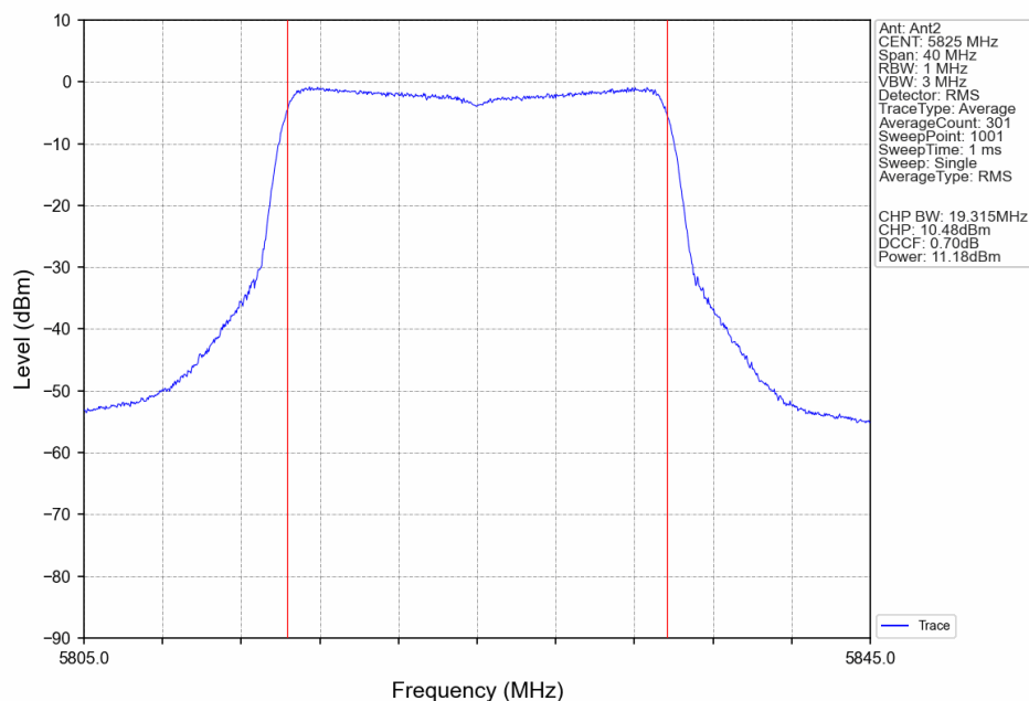
802.11ax(HEW20)_HCH_5825MHz_RU26_Left_Ant2_NTNV
