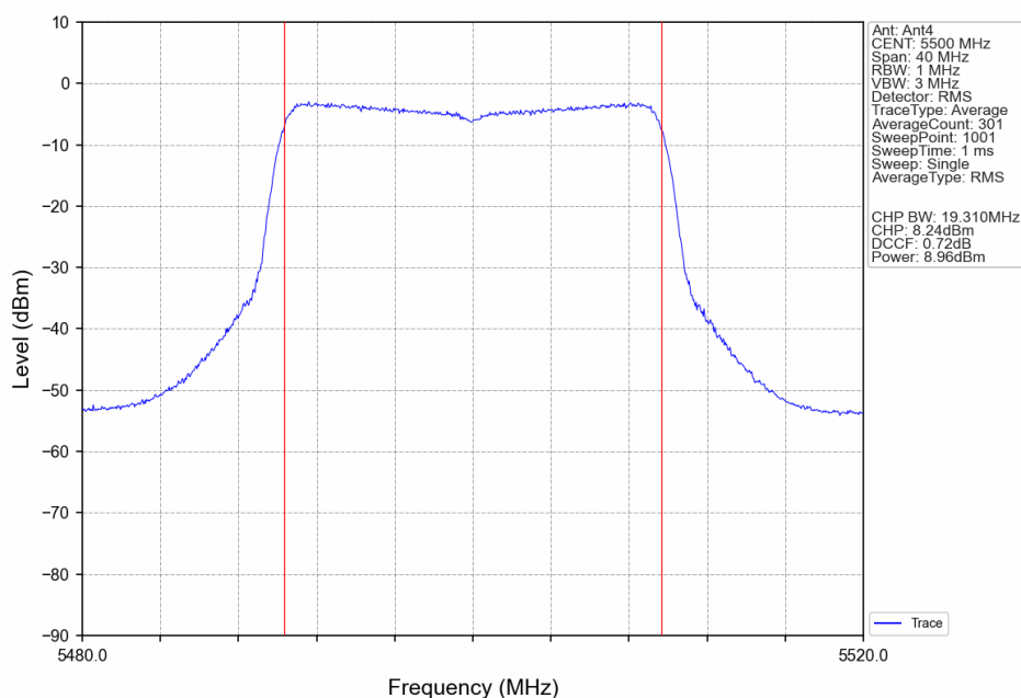
802.11ax(HEW20)_LCH_5500MHz_RU242_Left_Ant4_NTNV
