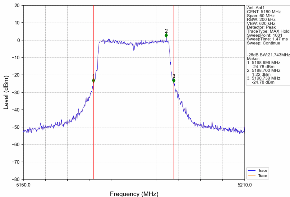
802.11ax(HEW20)_LCH_5180MHz_RU242_Left_Ant1_NTNV
