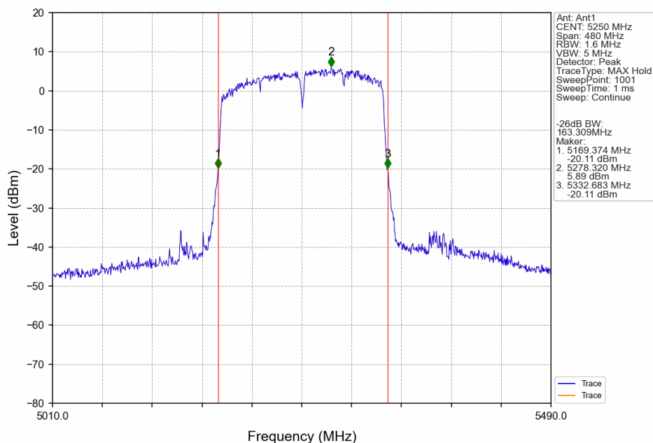
802.11ax(HEW160)_MCH_5250MHz_2xRU996_Left_Ant1_NTNV
