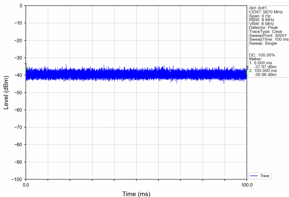
802.11ax(HEW40)_HCH_5670MHz_RU484_Left_Ant1_NTNV
