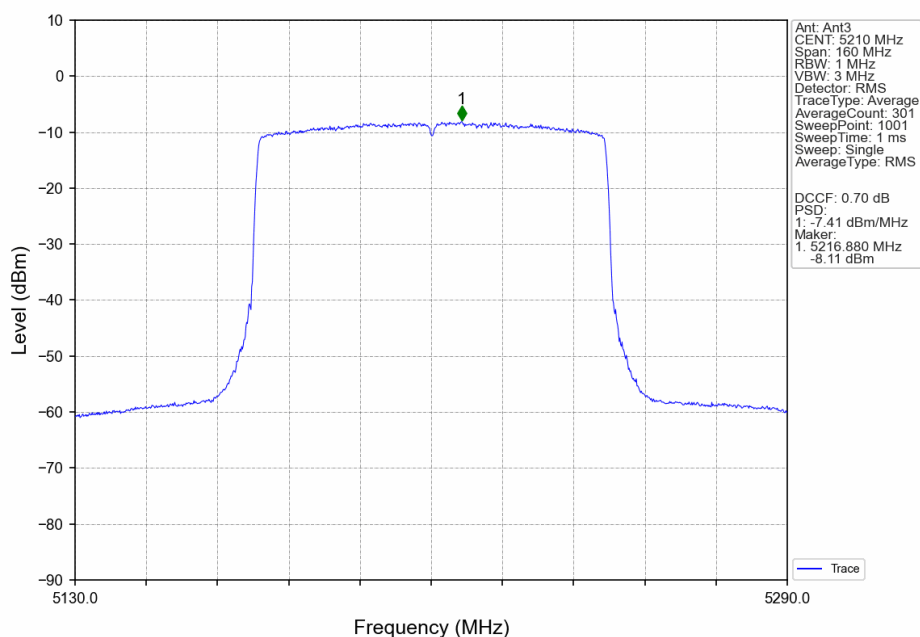
802.11ax(HEW80)_MCH_5210MHz_RU996_Left_Ant3_NTNV
