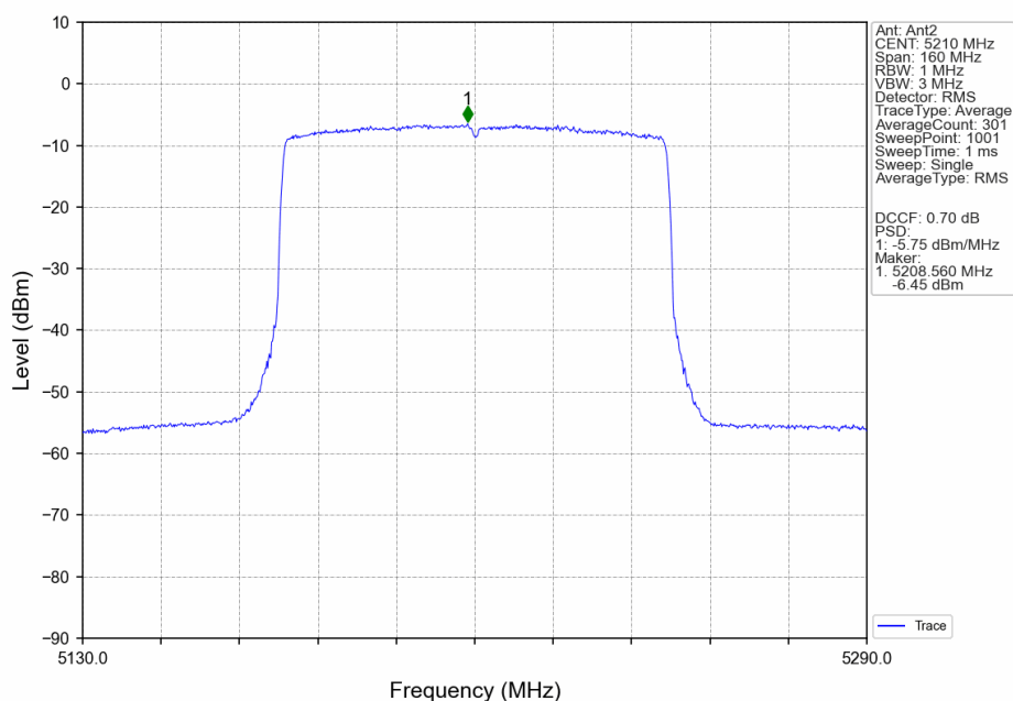
802.11ax(HEW80)_MCH_5210MHz_RU26_Left_Ant2_NTNV
