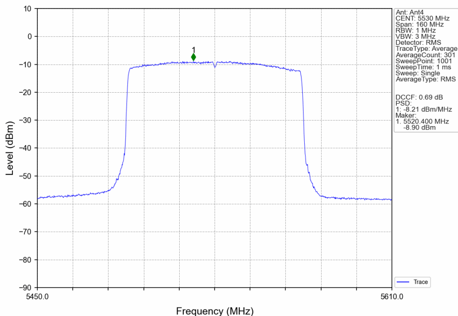
802.11ax(HEW80)_LCH_5530MHz_RU996_Left_MIMO_NTNV
