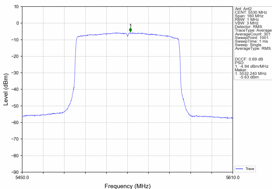
802.11ax(HEW80)_LCH_5530MHz_RU26_Left_Ant2_NTNV
