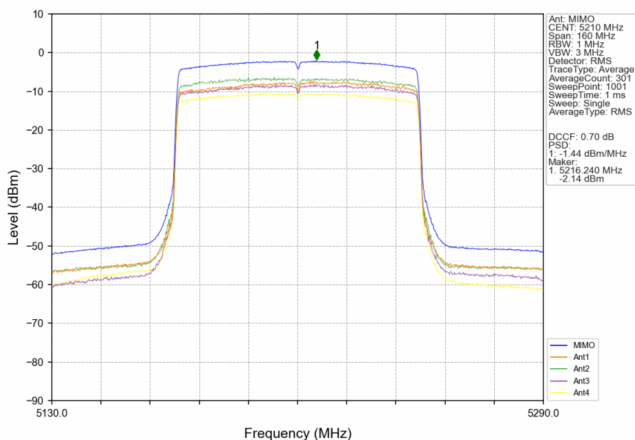
802.11ax(HEW80)_MCH_5210MHz_RU26_Mid_MIMO_NTNV
