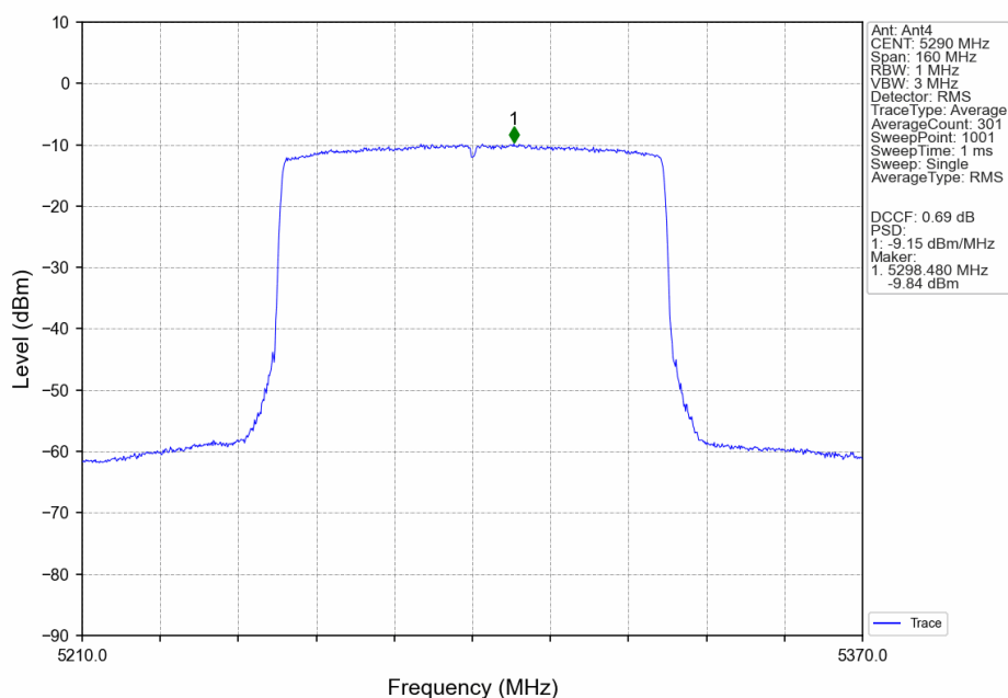
802.11ax(HEW80)_MCH_5290MHz_RU26_Left_Ant4_NTNV
