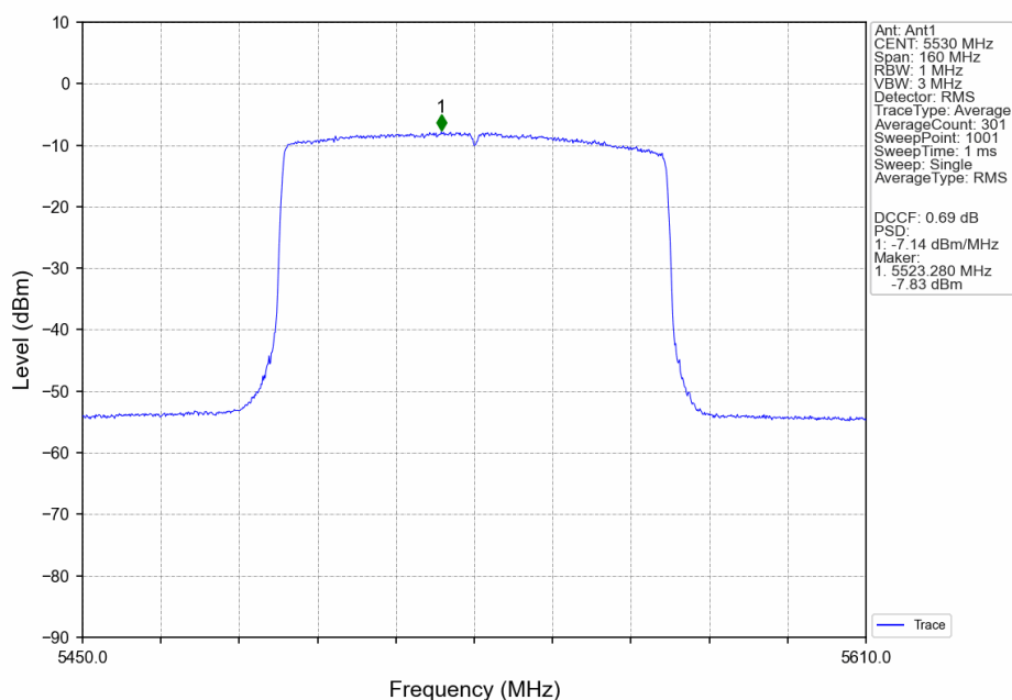
802.11ax(HEW80)_LCH_5530MHz_RU26_Mid_Ant1_NTNV
