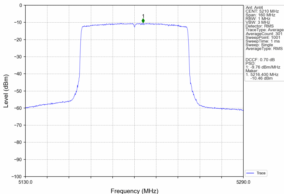
802.11ax(HEW80)_MCH_5210MHz_RU996_Left_MIMO_NTNV
