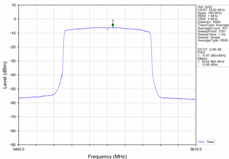
802.11ax(HEW80)_LCH_5530MHz_RU26_Right_Ant2_NTNV
